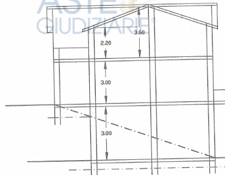
Sezione B-B
