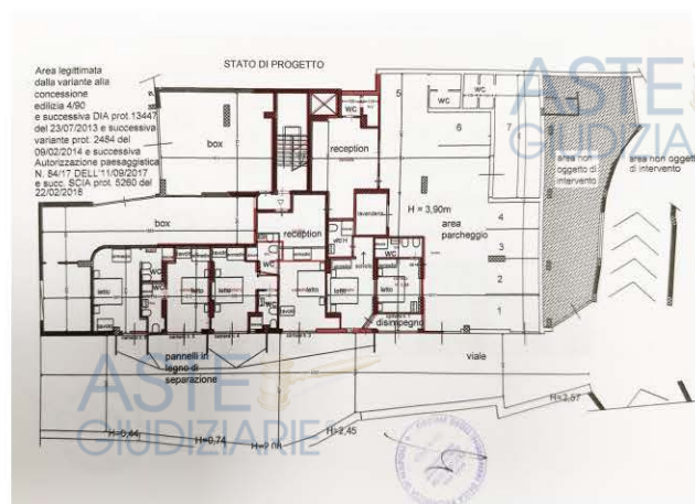
Sovrapposizione con lo stato di fatto
