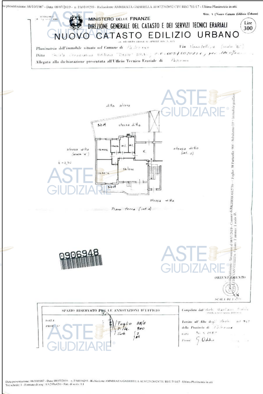
Planimetria catastale presentata il 06/10/1987 – Allegato 5
