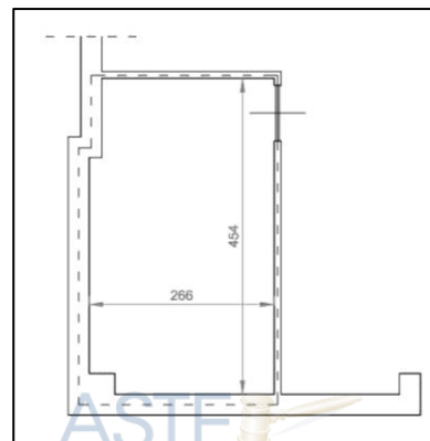
Planimetria stato di fatto locale cantina - Allegato 9
