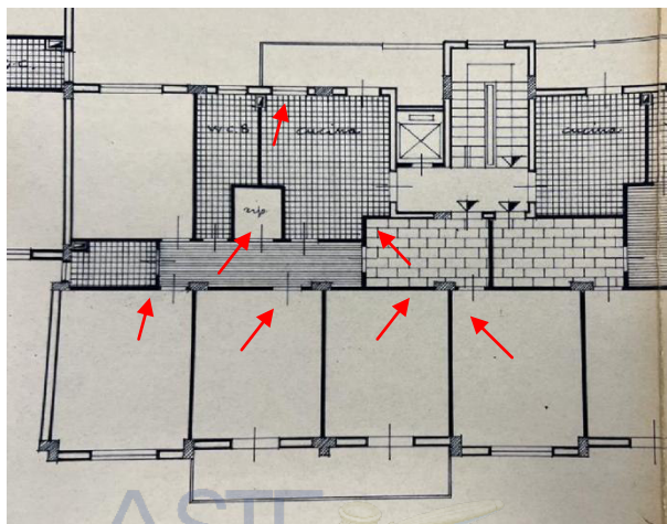
Planimetria di progetto
