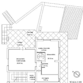
PIANO RIALZATO
