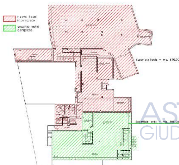
PIANTA PIANO SEMINTERATO STATO DI FATTO
