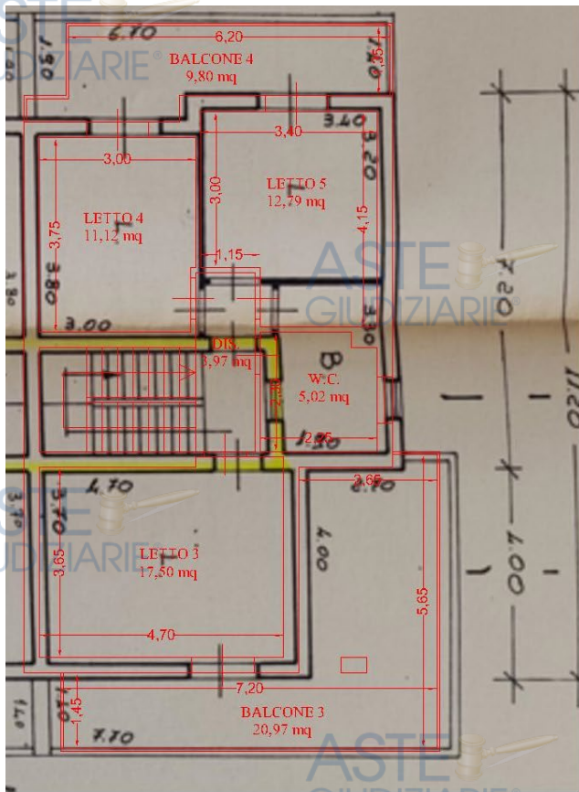
PIANTA PIANO SECONDO H=2,75m
