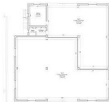
Stato di fatto
