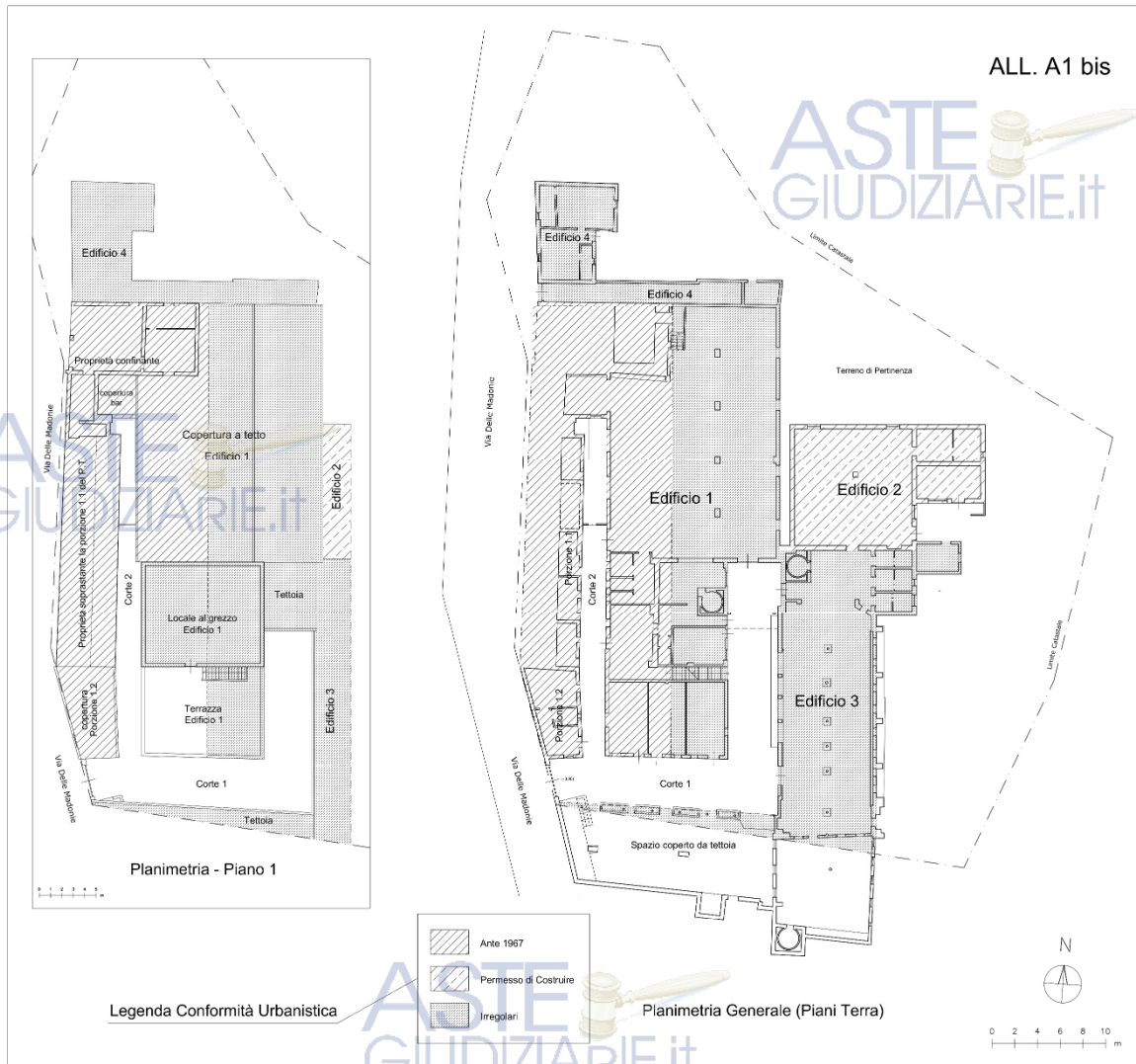
Figura 2: Planimetria dello stato dei luoghi con indicazione grafica delle difformità.
