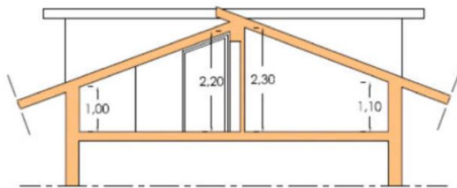
SEZIONE A-A'
