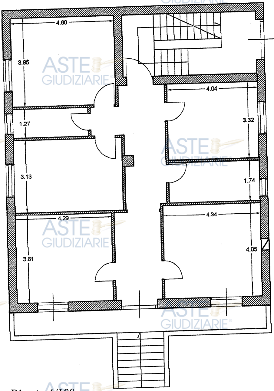
Pianta 1/100
