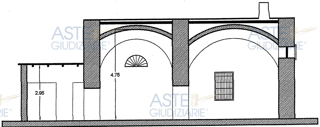
Sez A-A' 1/100
