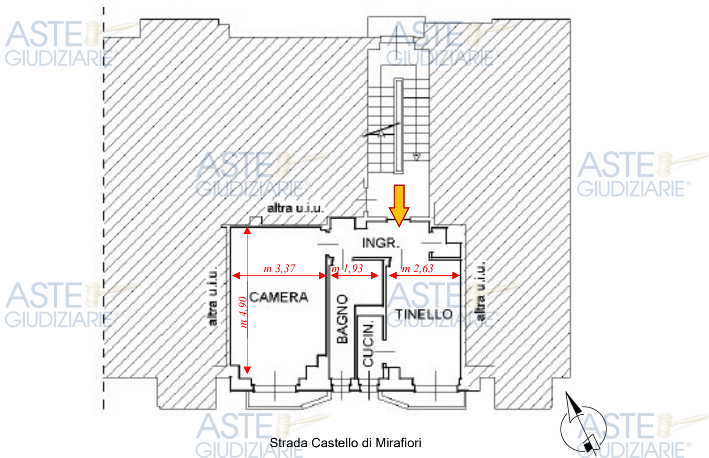
Planimetria non in scala dell'immobile pignorato (all. n. 3)
