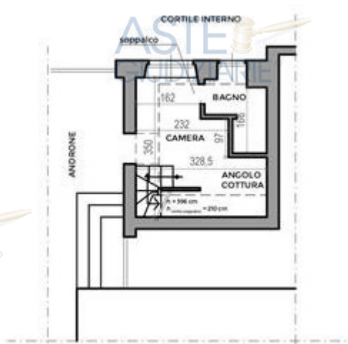
Rilievo qualitativo, indicativo dello stato dei luoghi
