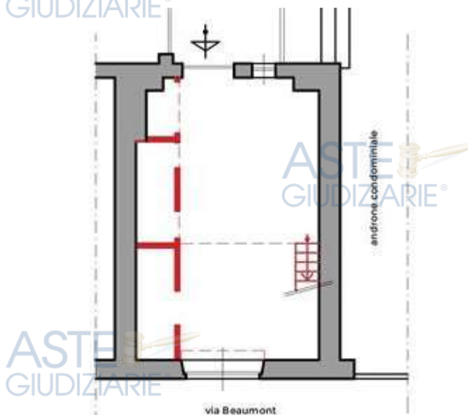
Sovrapposizione dello stato di fatto alla planimetria catastale in cui in rosso si rappresenta il costruito
