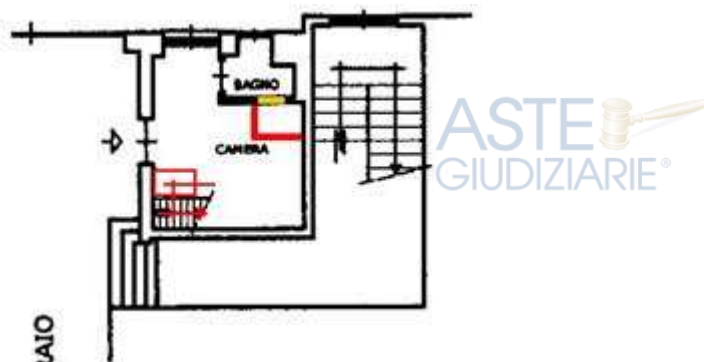
Sovrapposizione qualitativa dello stato di fatto alla planimetria catastale in cui in rosso si indicato le nuove costruzioni e in giallo le demolizioni rispetto allo stato autorizzato
