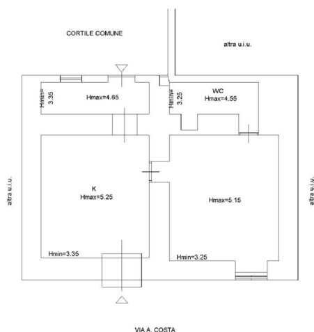
Planimetria catastale
