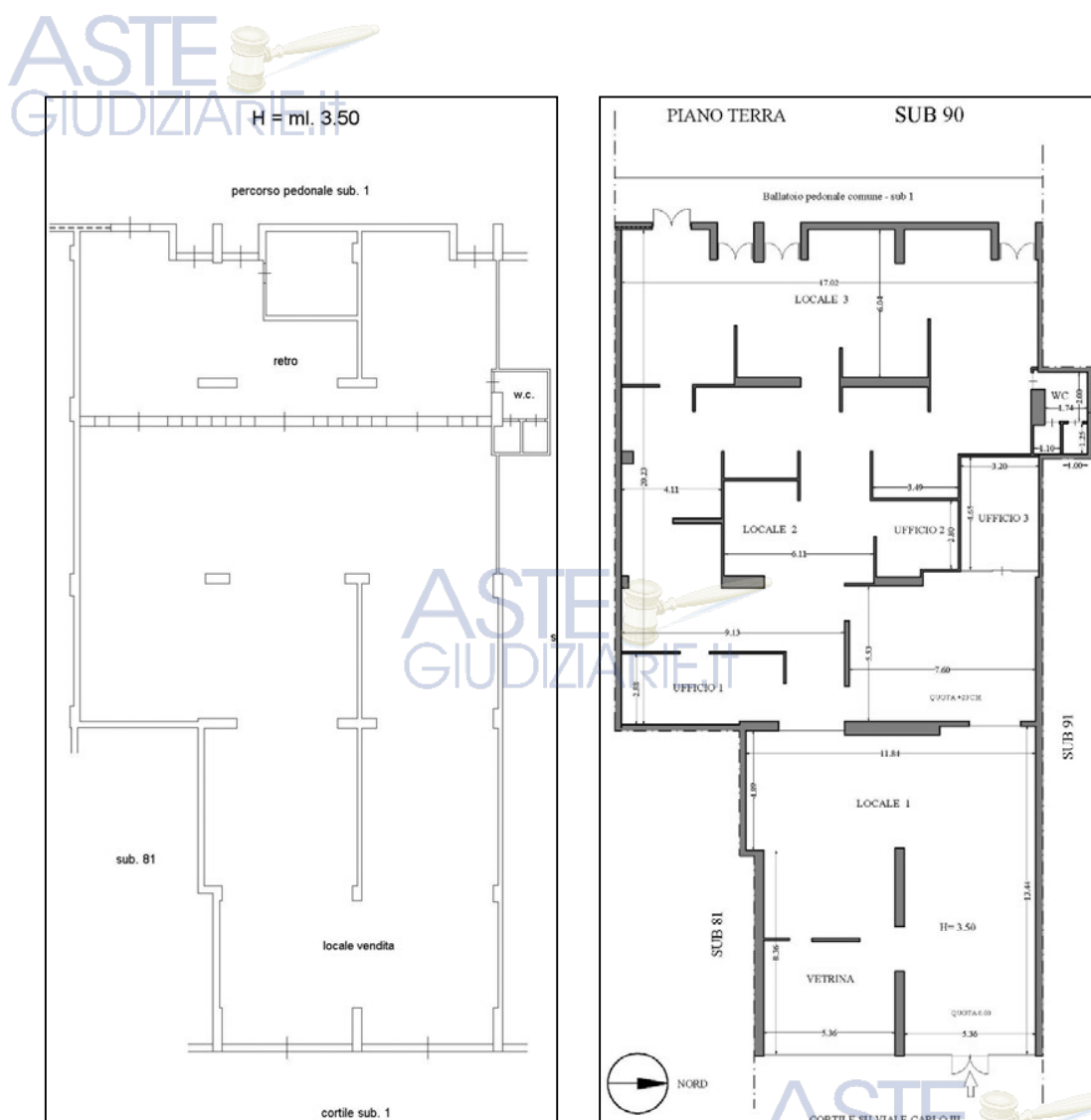
Fig. 5 – Confronto delle Planimetrie in atti al Catasto con lo stato dei luoghi - NON CONFORME
