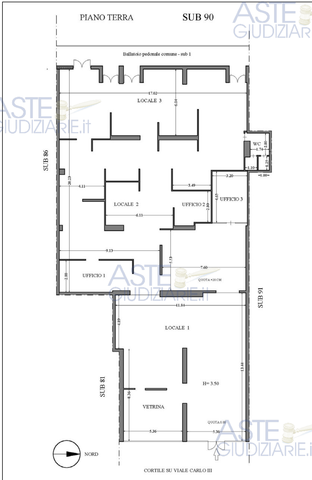
Fig. 2 - Pianta dello stato dei luoghi
