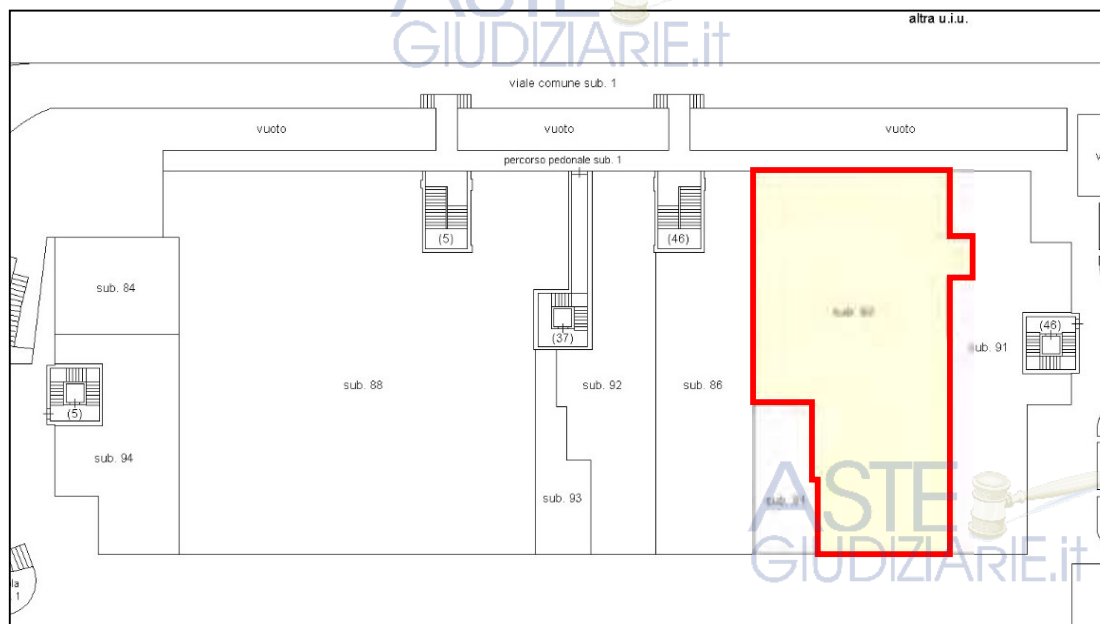
Fig. 3 – Elaborato planimetrico con individuazione LOTTO N. 39
