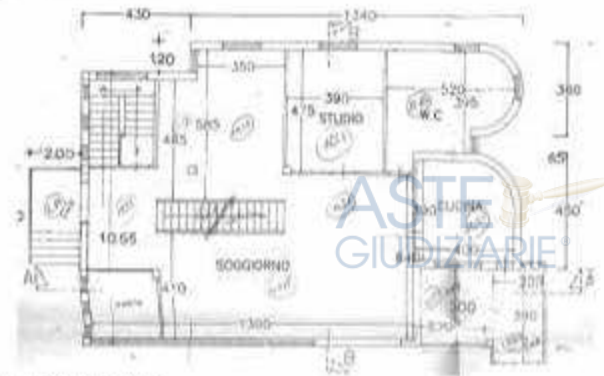
PIANTA PIANO REALZATO
