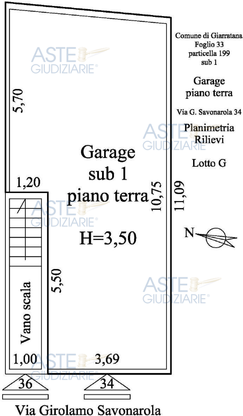
Figura 6 Lotto G – Rilievi piano terra Foglio 33 Giarratana particella 199 sub 1
