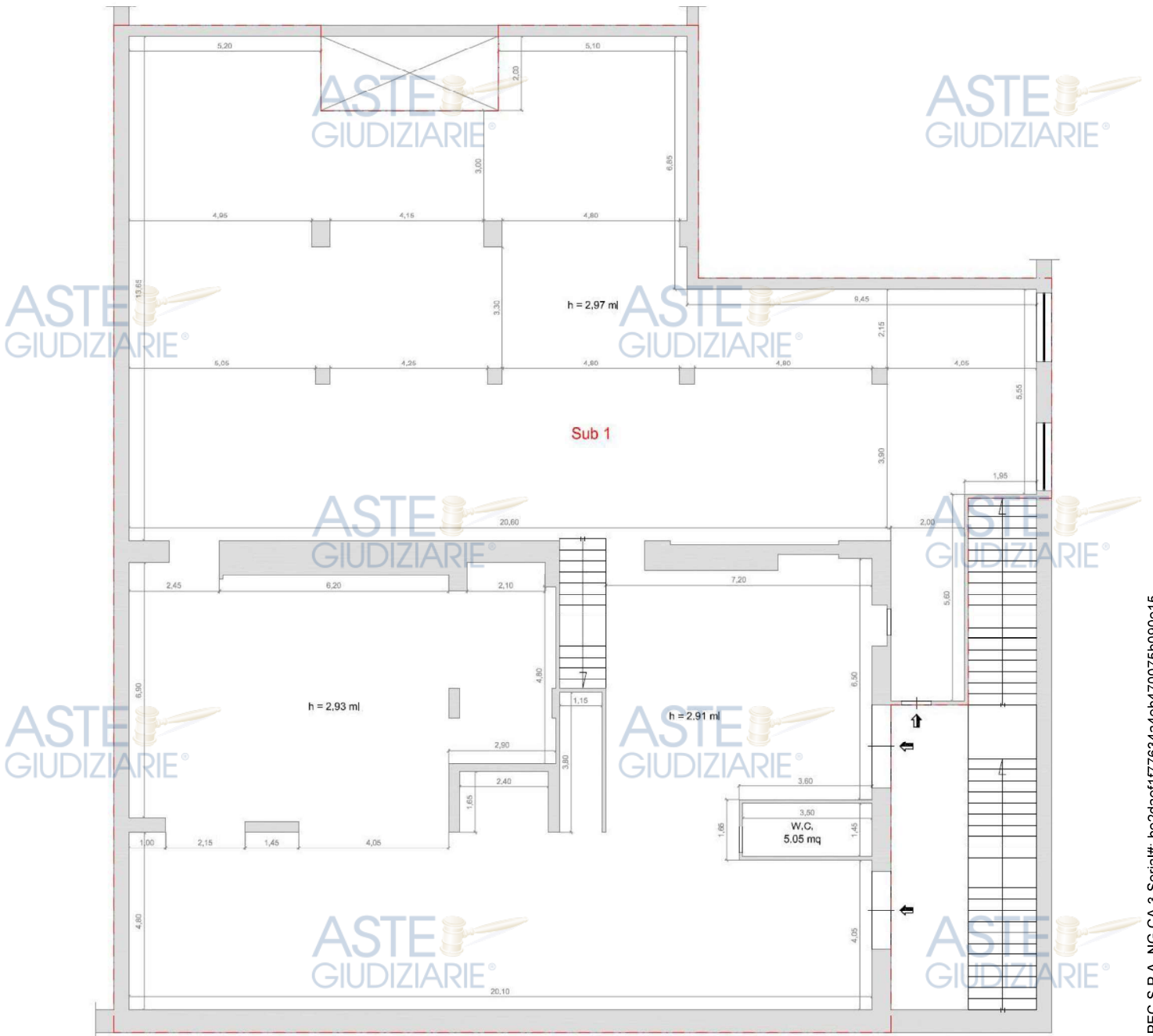
Figura 3 - Planimetria Catastale Immobile Pignorato, Piano Seminterrato, Foglio 48, p.lla 76, Sub 1.
