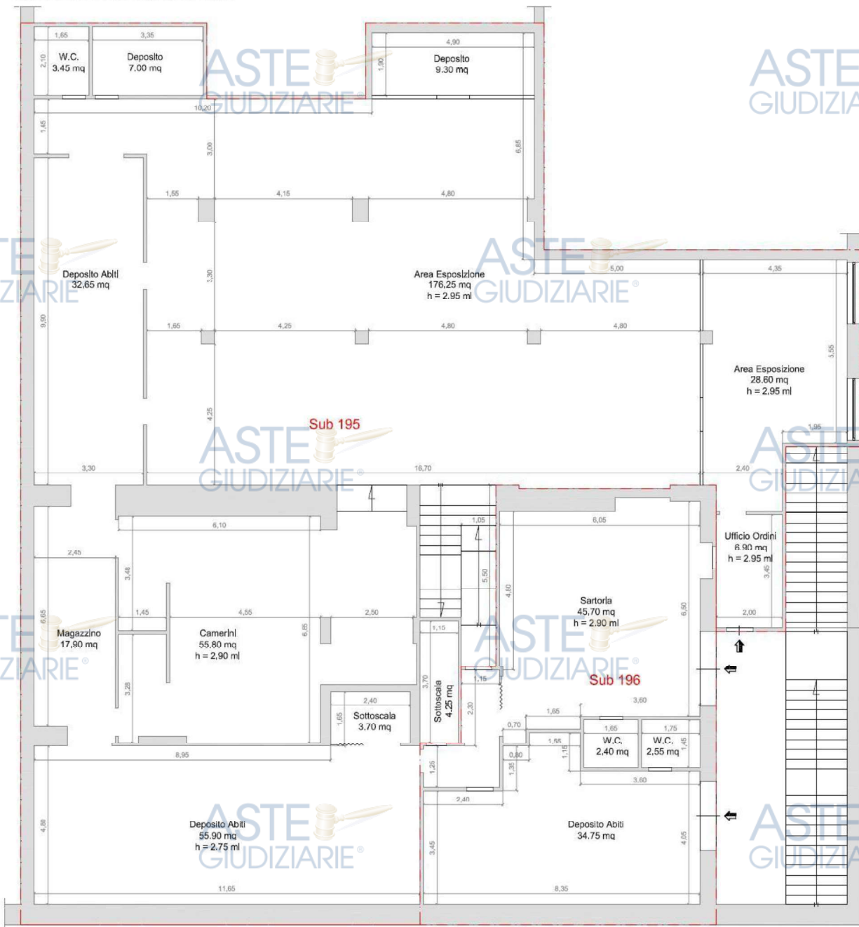
Figura 7 - Planimetria Stato di Fatto Piano Seminterrato, Foglio 48, p.lla 76, Sub 195-196 (Ex Sub 1).
