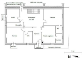
Figura 7 - Planimetria dello stato reale dei luoghi - Piano 1° (appartamento)
