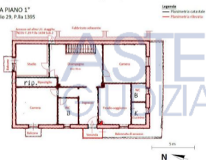
Figura 12 - Sovrapposizione planimetria dello stato reale dei luoghi con la planimetria catastale - Piano 1°
