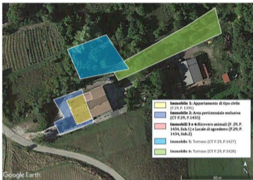
Figura 10 - Ortofoto con individuazione planimetrica dei beni staggiti
