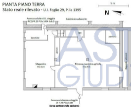
Figura 6 - Planimetria dello stato reale dei luoghi - Piano Terra (magazzino e rimessa macchine agricole)
