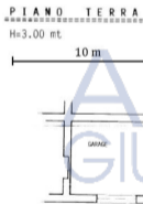
Figure 2 - Estretto Planimetria Catastale - Autorimessa (Ricovero Animali) NCEU Foglio 29, Part. 1434 sub. 1
