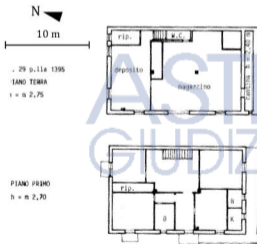
Figura 1 - Estratto Planimetria Catastale - Abitazione di tipo civile NCEU Foglio 29, Particella 1395
