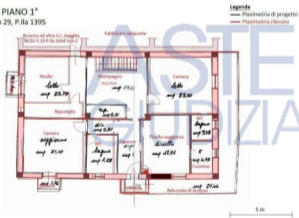
Figura 18 - Sovrapposizione stato reale dei luoghi e progetto autorizzato - Planimetria Piano 1°
