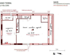
Figura 17 - Sovrapposizione stato reale dei luoghi e progetto autorizzato - Planimetria Piano Terra
