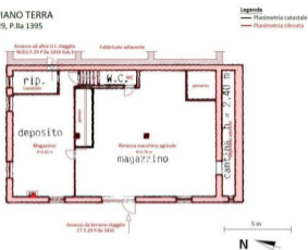
Figura 11 - Sovrapposizione planimetria dello stato reale dei luoghi con la planimetria catastale - Piano Terra
