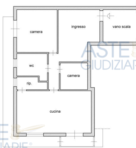
PIANTA DELLO STATO DI FATTO
