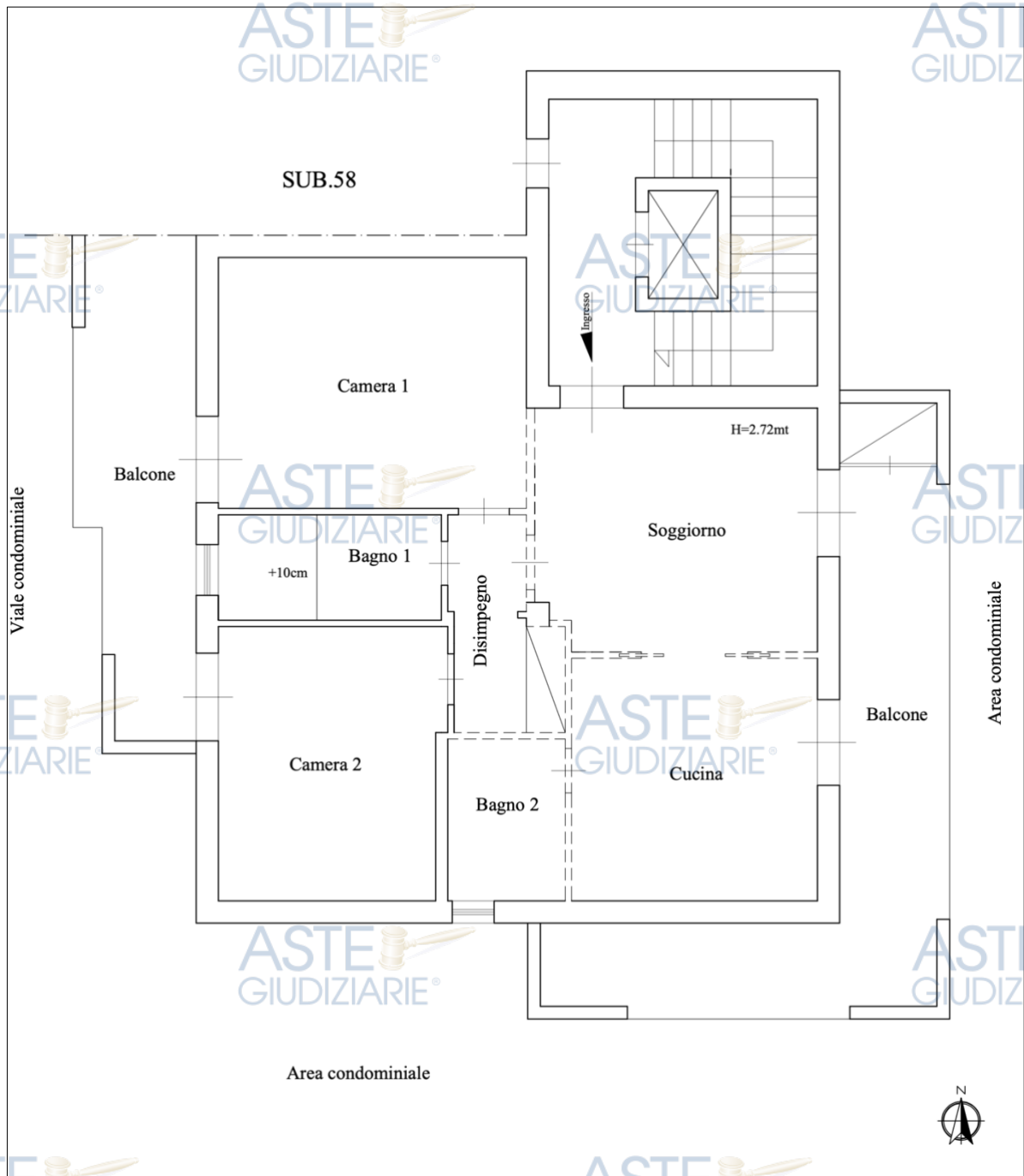
Figura 6 - Grafico difformità catastale
