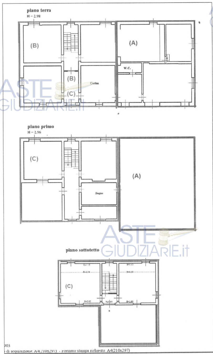
Ipotesi divisionale - Planimetrie P.T. (A), P. 1° (B), Sottotetto (C).
