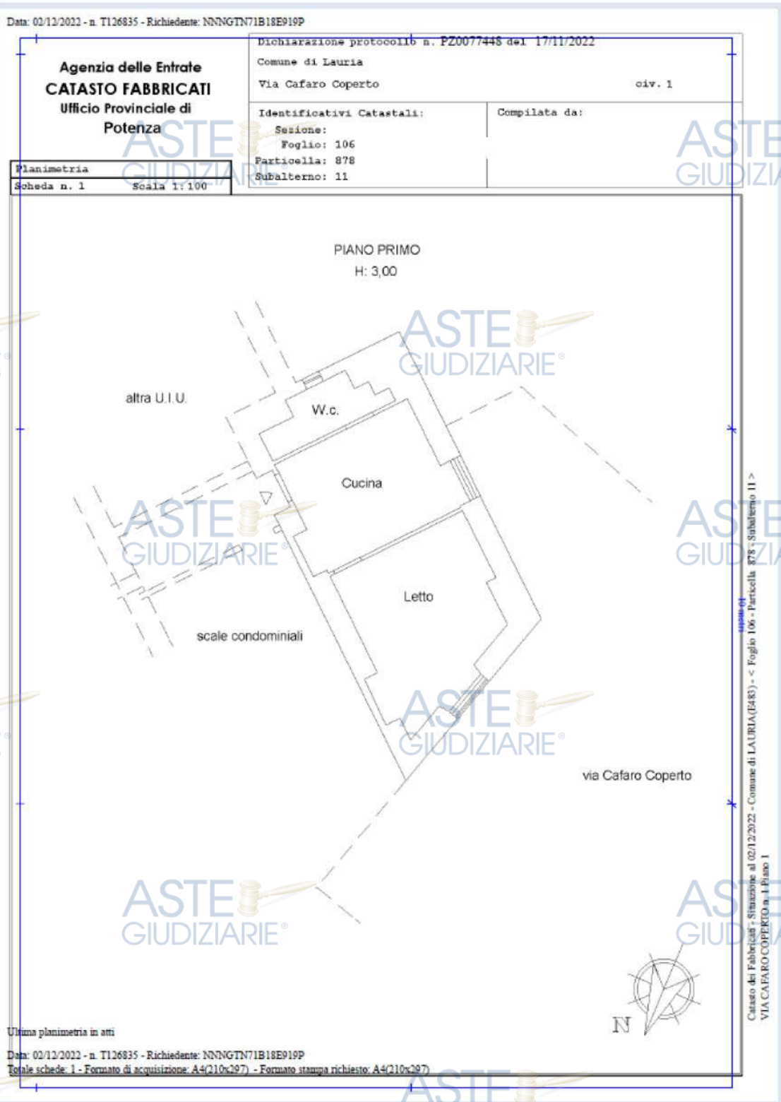
Fig. 10 – Planimetria “aggiornata” Unità Fg. 106 P.IIa 878 sub. 11
