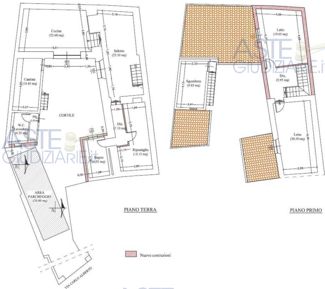
Pianta del piano terra e del piano primo estratte dalla tavola 2 di progetto (CE n°41/2010)
