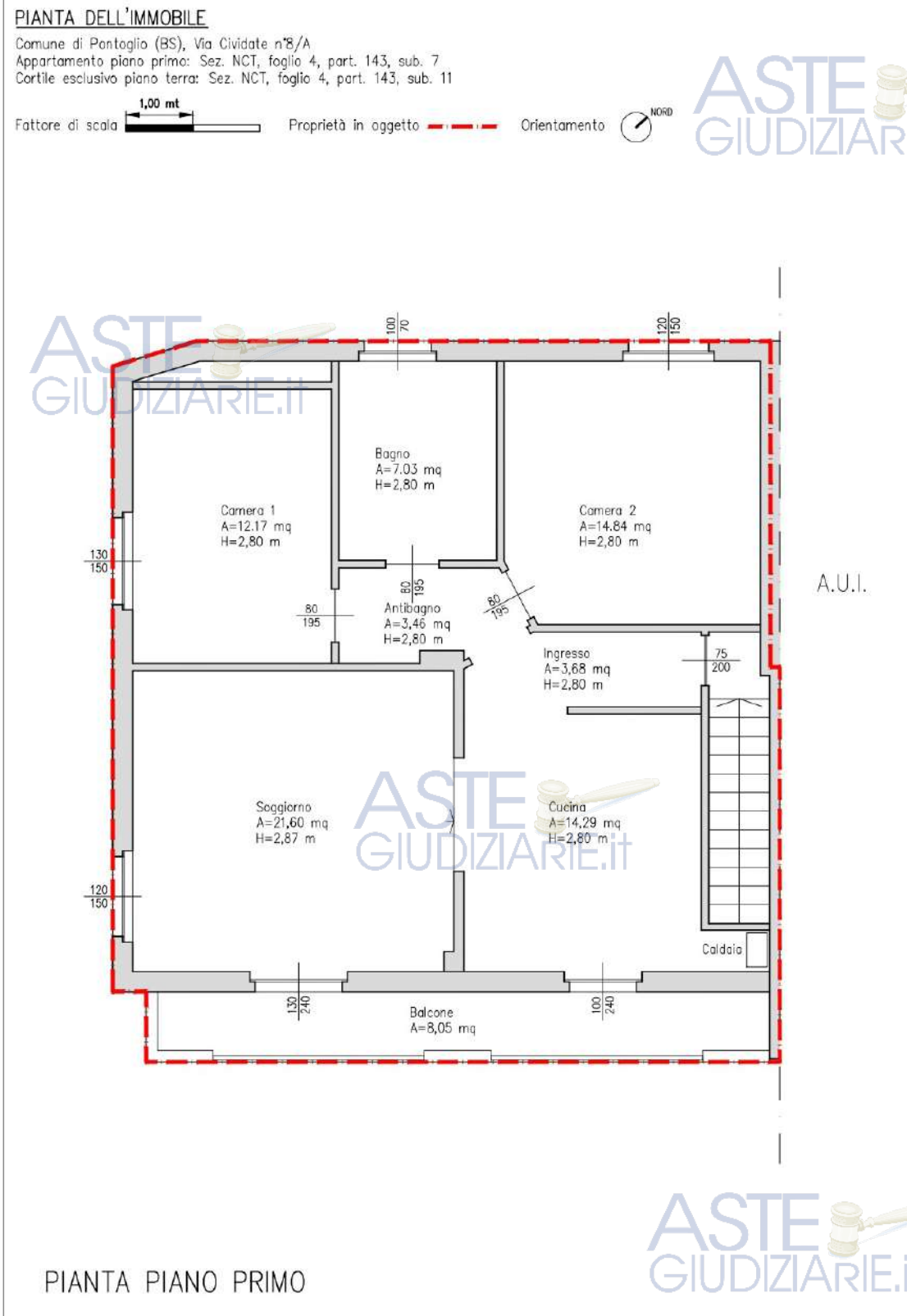
Figura 08: Pianta piano primo
