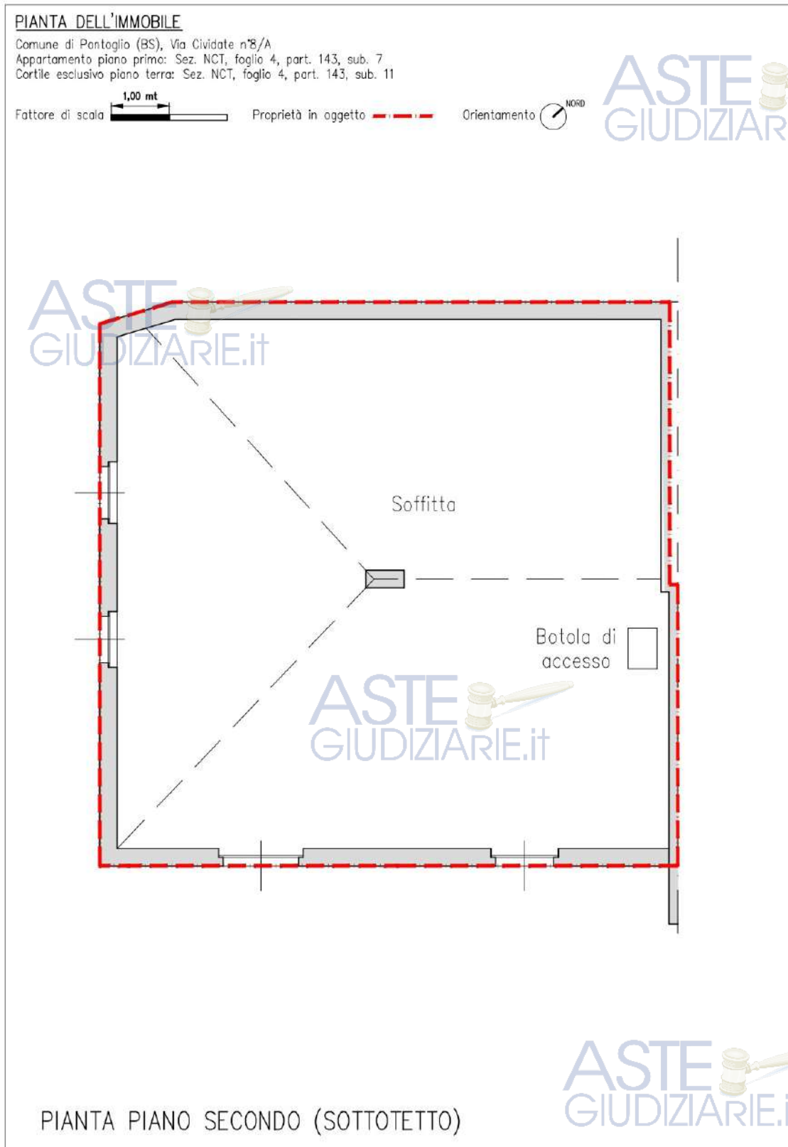
Figura 09: Pianta piano secondo (sottotetto)
