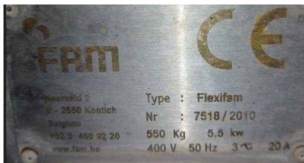
Foto 38 - Targhetta Cubettatrice FAM
