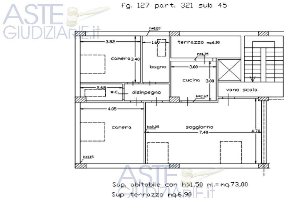
PIANTA PIANO QUARTO mansardato fg. 127 part. 321 sub 45
