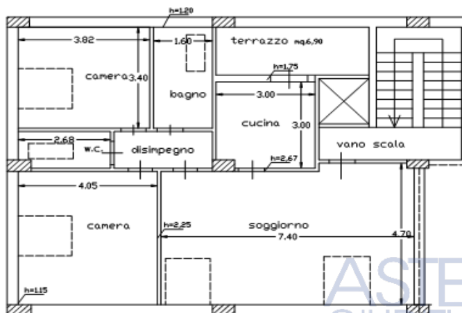
PIANTA PIANO QUARTO mansardato fg. 127 part. 321 sub 45
