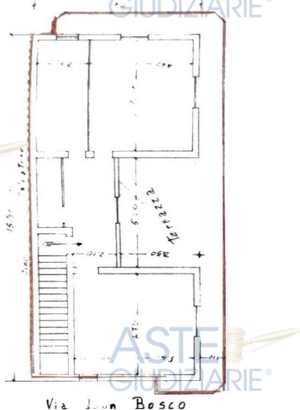
Plan Piano secondo Progetto C.E. del 08/09/1984
