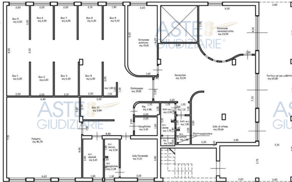
Pianta piano terra – scala 1:200
